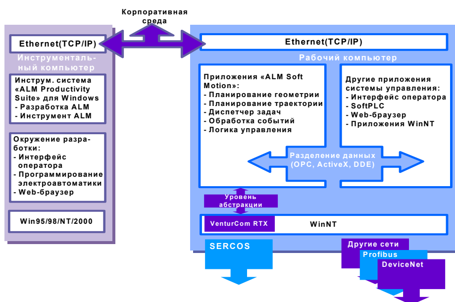
Рис.3. Подсистема Motion Control.
