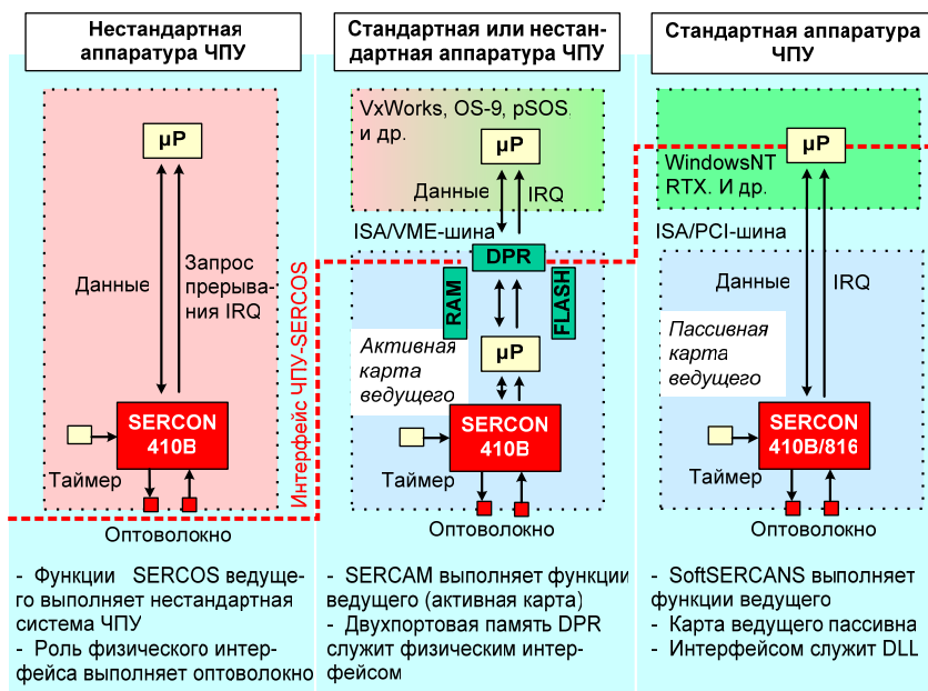
Рис.8. Переход от SERCANS к SoftSERCANS.
