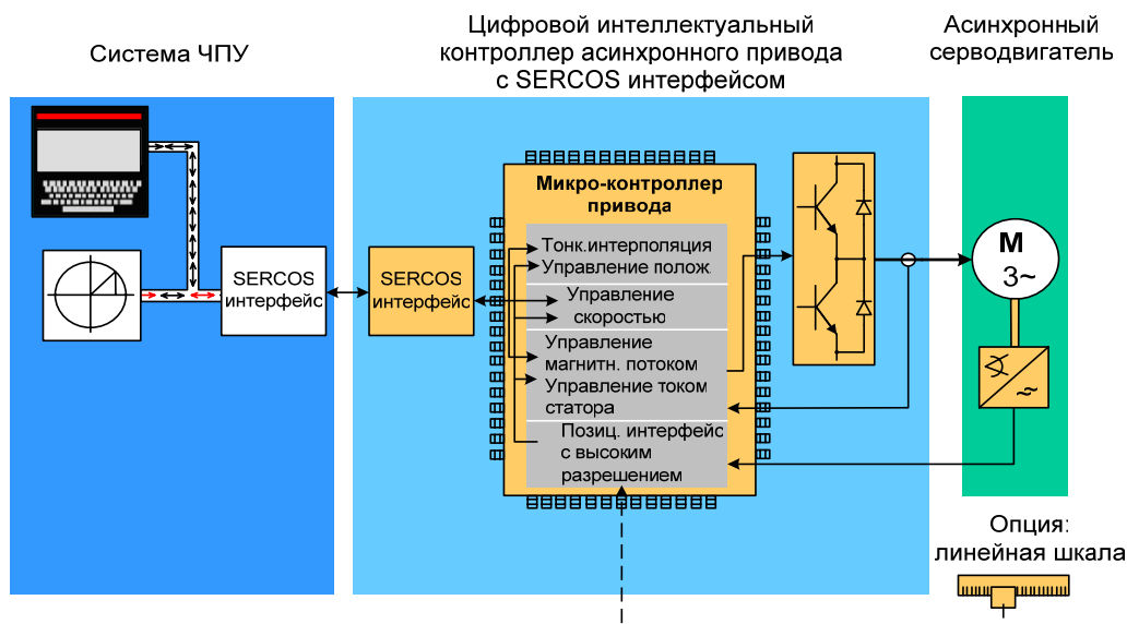
Рис.7. SERCOS интерфейс систем ЧПУ
