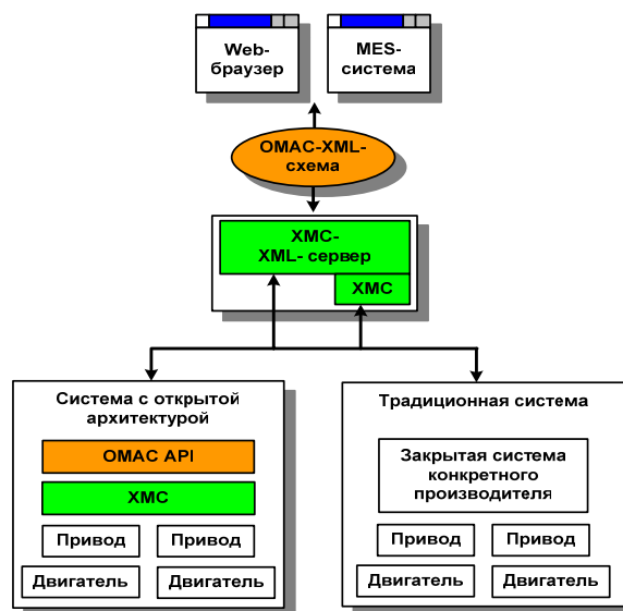
Рис.4. Система ЧПУ с Web-доступом.
