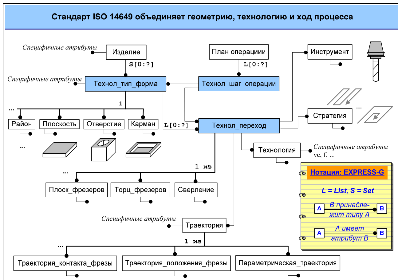
Рис.5. Управляющая информация в стандарте ISO 14649.
