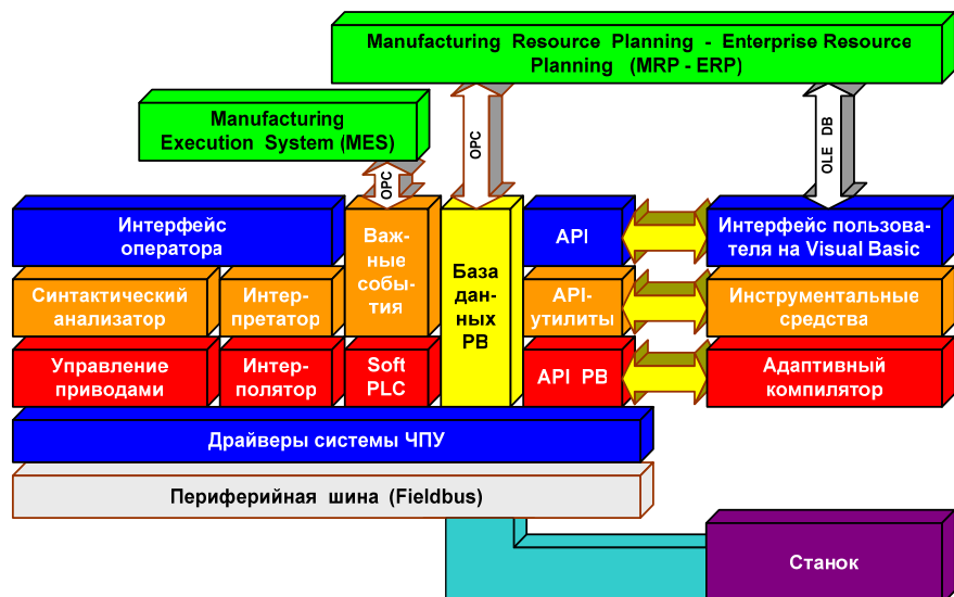
Рис.2. Пример архитектуры открытой системы ЧПУ OpenCNC.
