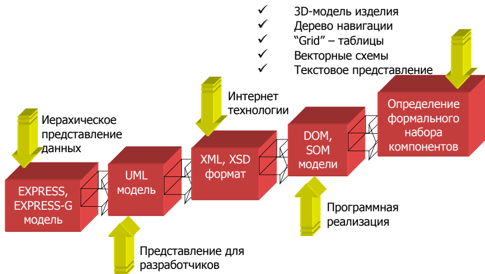
Рис.13. Трансформация моделей STEP-NC.
