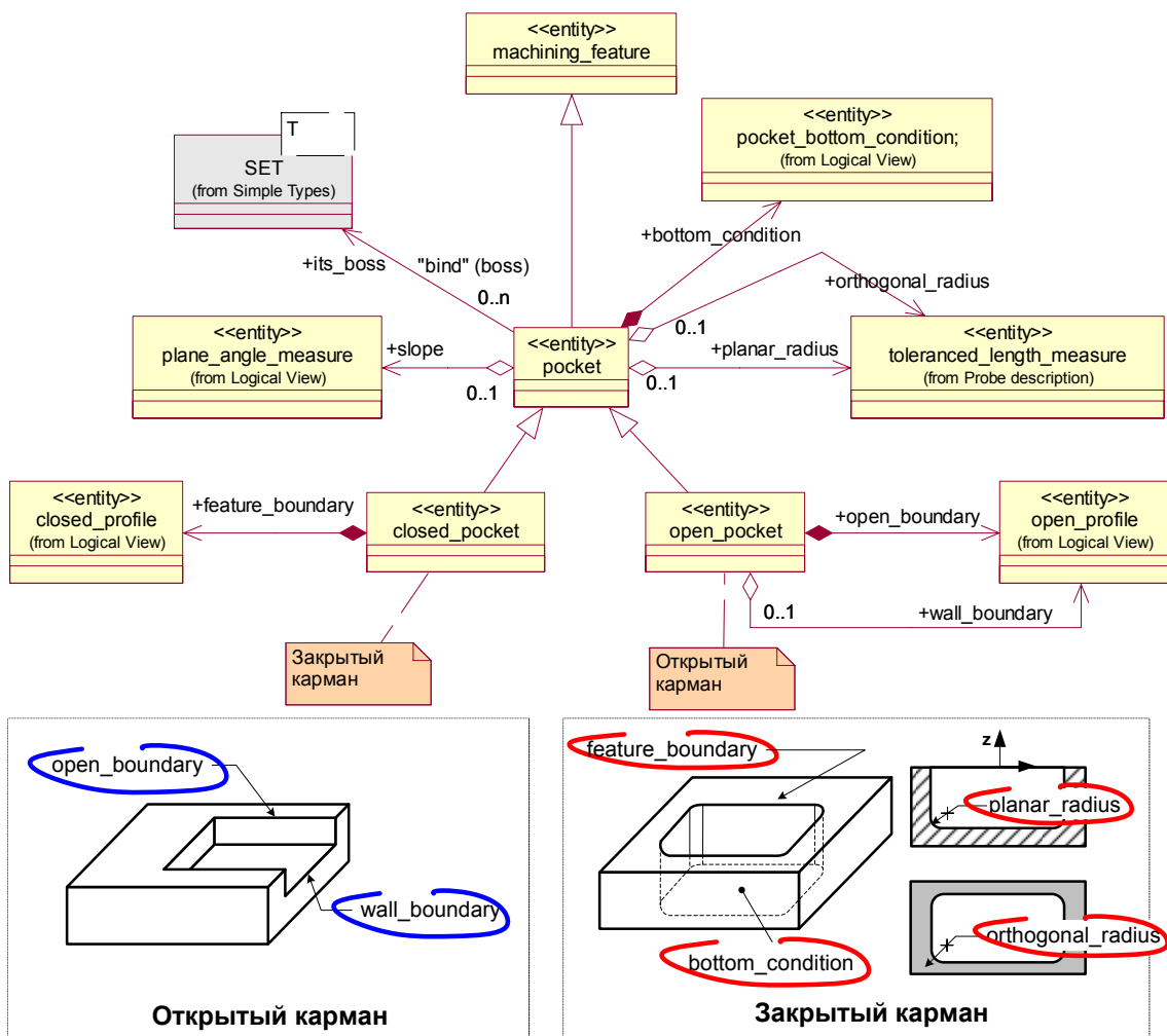
Рис.14. Фаза UML модели STEP-NC.
