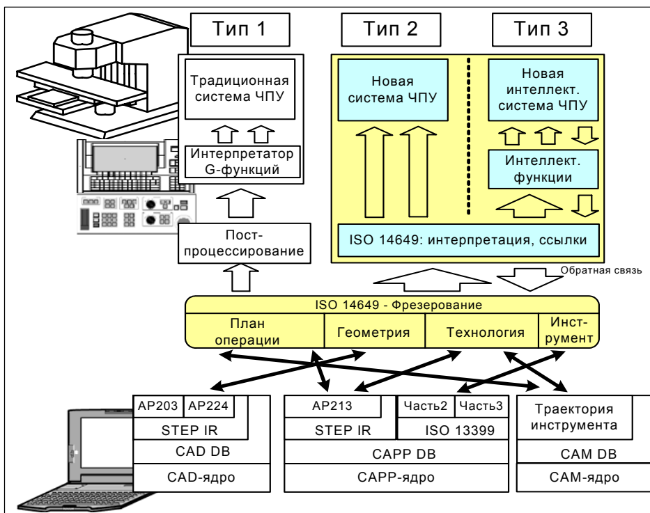
Рис.6. Системы ЧПУ, воспринимающие стандарт STEP-NC
