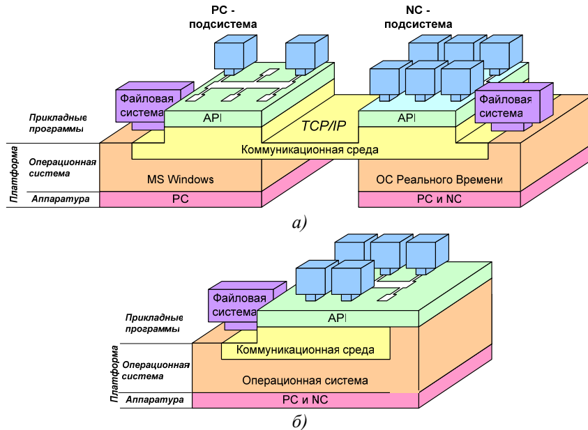
Рис.1. Архитектурные варианты систем ЧПУ.
